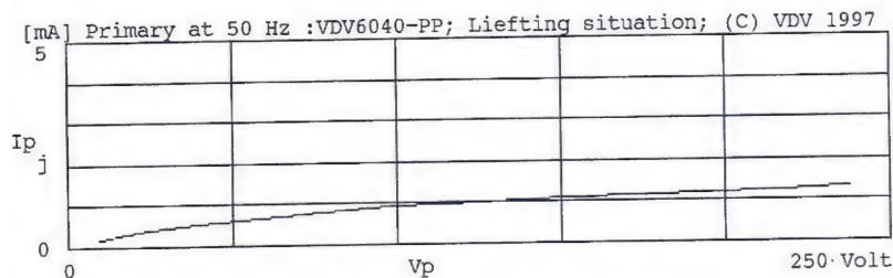
Figuur 3 50 Hz wisselstroom door en spanning over de gehele primaire wikkeling voor I_p bepaling.
